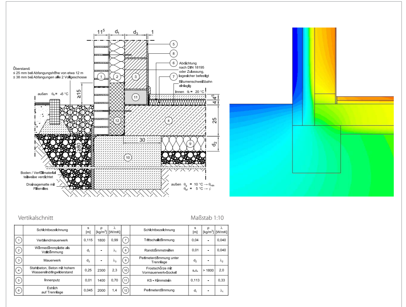
Abbildung 3: Wärmebrückenoptimiertes Sockelanschlussdetail und die dazugehörige Isotherme für zweischaliges Verblendmauerwerk bei einem nicht unterkellerten Gebäude (numerisch mit der Finiten-Elemente-Methode berechnet, Erläuterungen und weitere Beispiele auf der Homepage: www.ziegelindustrie.de ).
